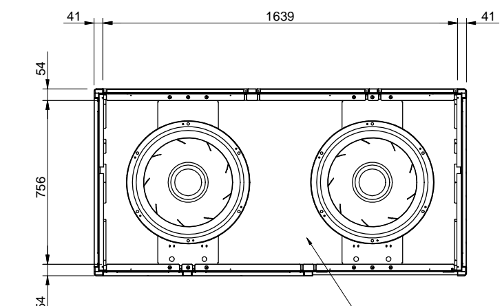
SEZIONE A-A
